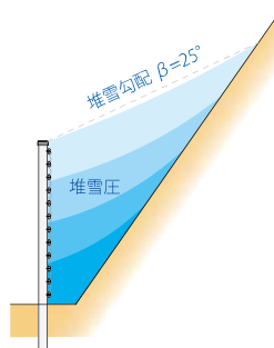
■ 施工事例 (せり出し防止柵)
