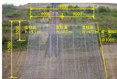
■ 実験供試体 (BRN-250~1300)
