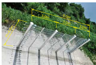
■ 実験供試体
