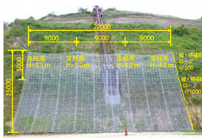
■ 実験供試体 (BRN-2100)
