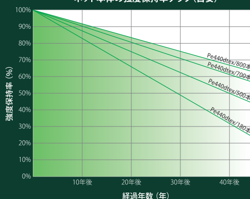
ネット本体の強度保持率グラフ(目安)
