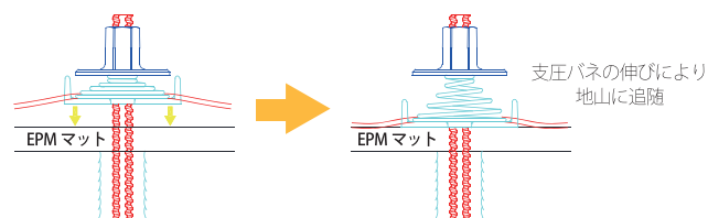
支圧バネの反発力による抑え込み効果 (植生基盤材の流出抑制効果)
