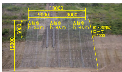
■ 実験供試体 (BRN250~BRN1300)
