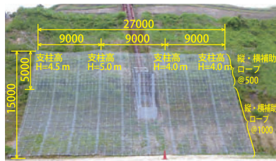
■ 実験供試体 (BRN2100)
