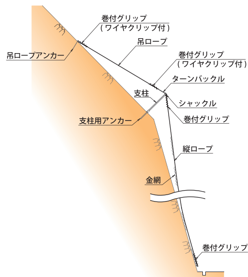
断面図
