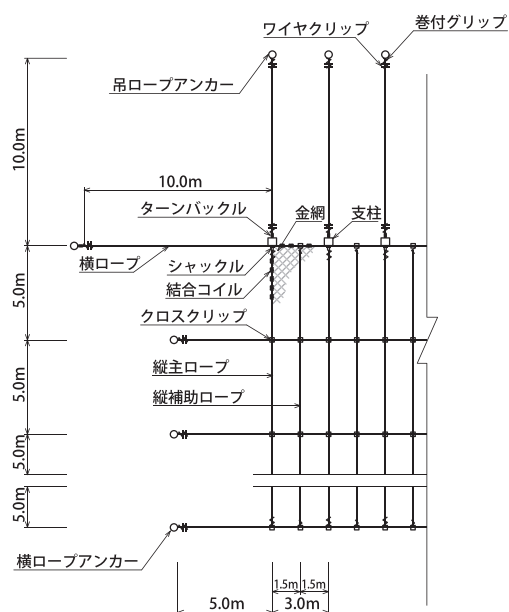
展開図
