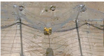
■ TYPE-100kJ重錘捕捉状況
