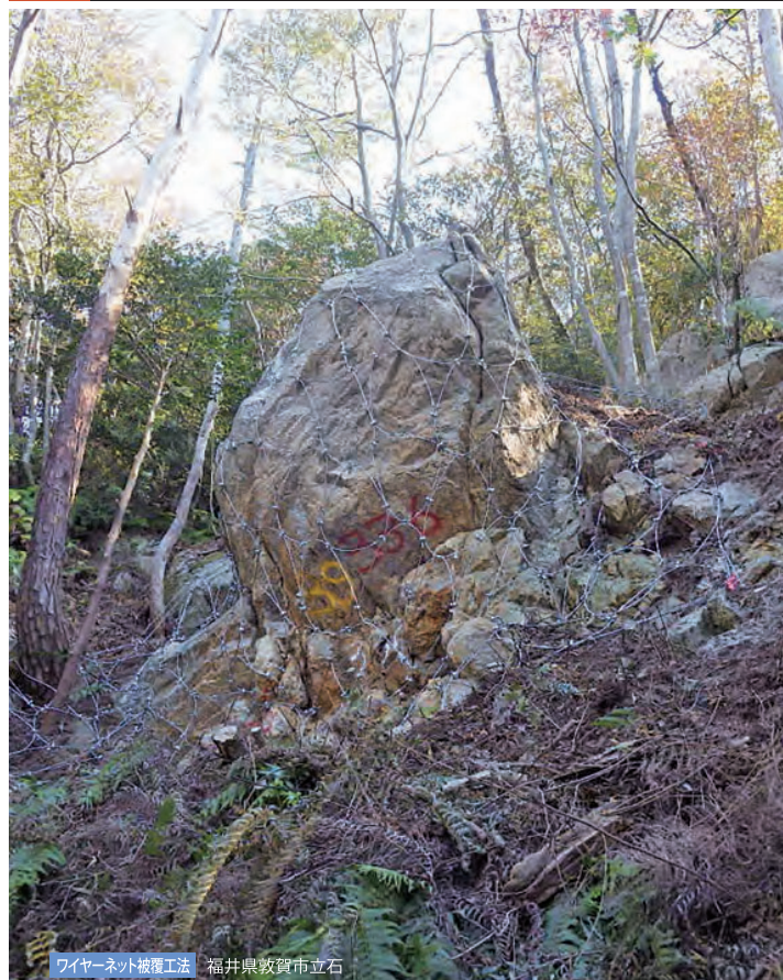
ワイヤーネット被覆工法 福井県敦賀市立石
