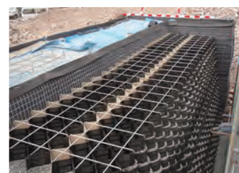
■ ジオセル(RGB-TW)
