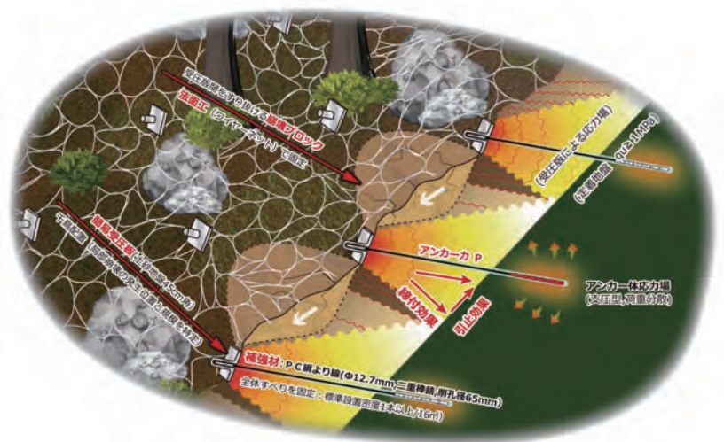
■ 抑止機構図
