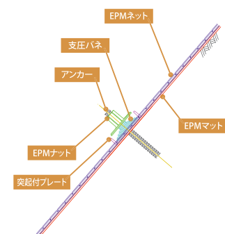
■ 各部材名称
