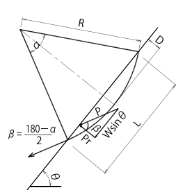
① すべり荷重の算定
