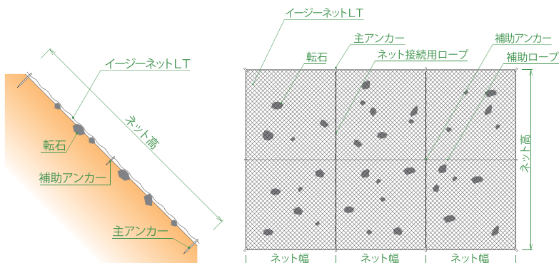
■ 施工事例 (イージーネットLT)
