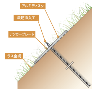
■ 各部材名称
