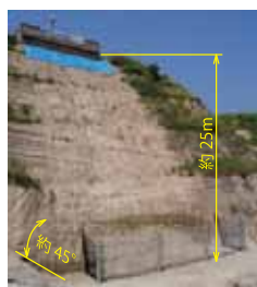
■ 実験状況 (土砂流下前)
