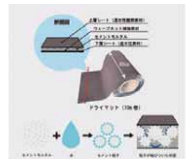
■ドライマット断面と固まるまでのプロセス
