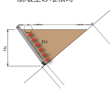
崩壊土砂堆積時
