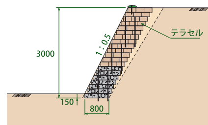
■ 各部材名称
