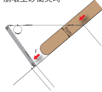
崩壊土砂衝突時
