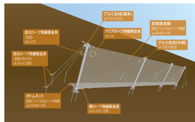
■ 各部材名称
