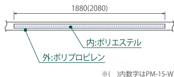
■ 吊ベルト (2重構造) 詳細図
