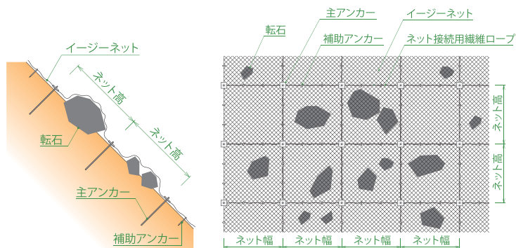
■ 施工事例 (カバータイプ)
