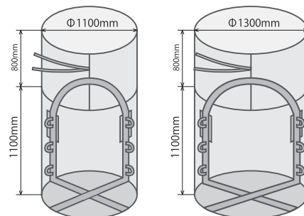
■ 構造図 (PM-15-N)
