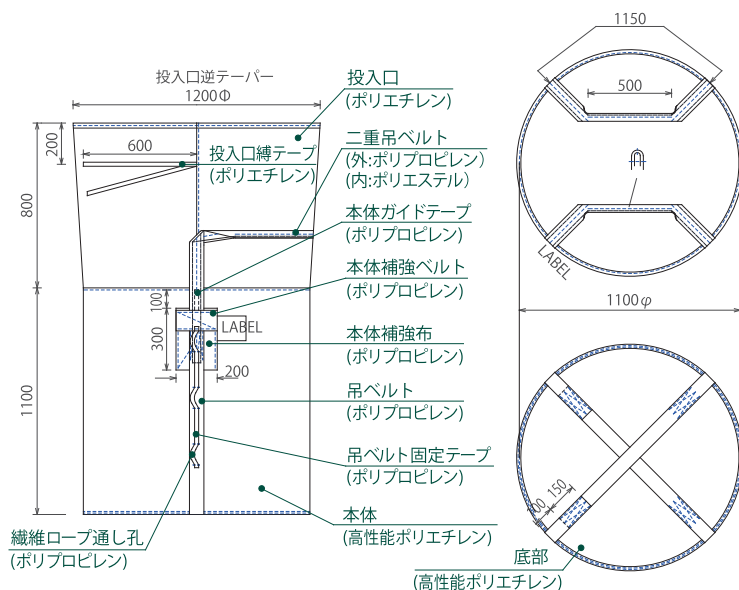
■ 大型土のう構造図 (PM-15-N)
