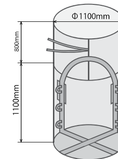
■ 構造図
