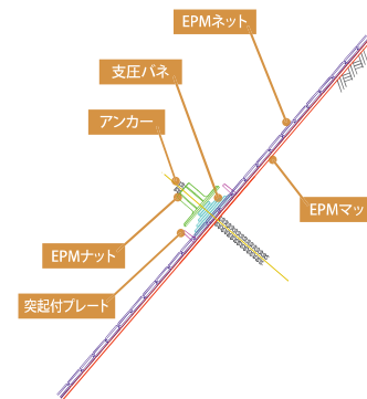
■ 各部材名称
