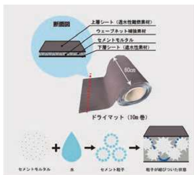
■ドライマット断面と固まるまでのプロセス
