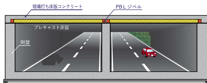
■ 断面イメージ
