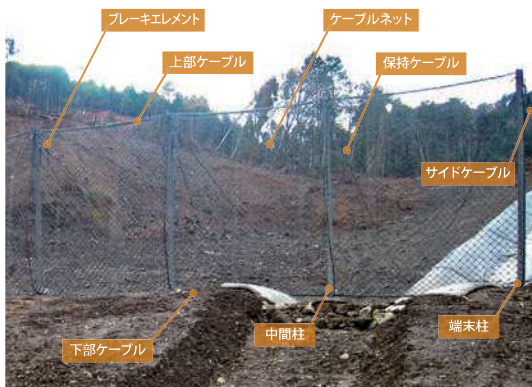
■ 各部材名称
