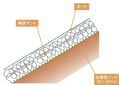
■ 各部材名称
