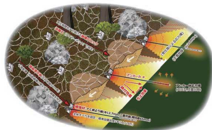
■ 抑制機構図
