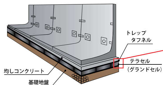
■ 構造イメージ
