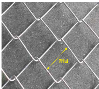
EPMネット -1 型 【材質：JISG3505】
