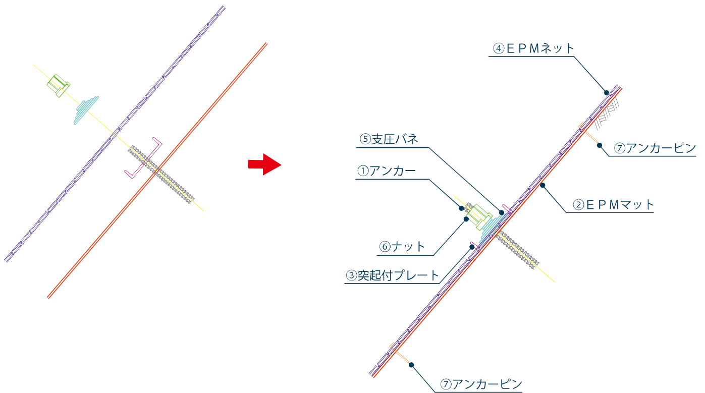
【 A 部断面図 】
