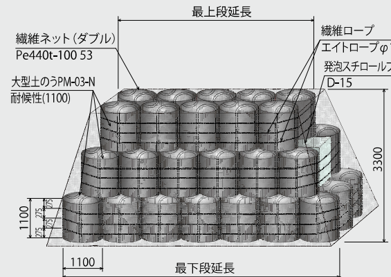
正面図
